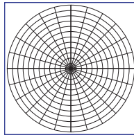
Polar Coordinates
